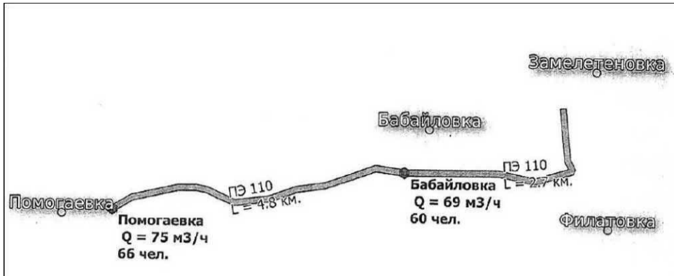
Рис. 3 Межпоселковый газопровод от с. Замелетеновка до д. Бабайловка и д. Помогаевка Любинского района Омской области
