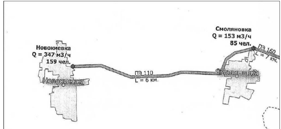
Рис. 8 Межпоселковый газопровод от д. Смоляновка до с. Новокиевка Любинского района Омской области
